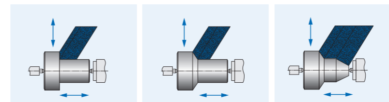
SCHRÄGEINSTICH-AUSSENRUNDSCHLEIFEN MIT EJ 11, EJ 31 UND EJ 51
